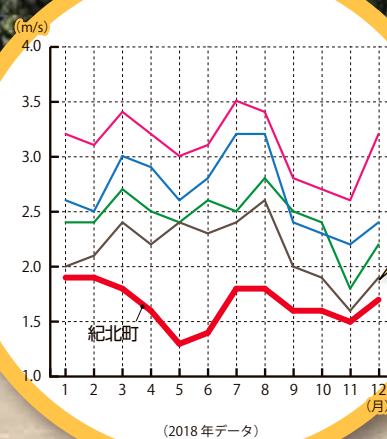
風速の平均値グラフ
