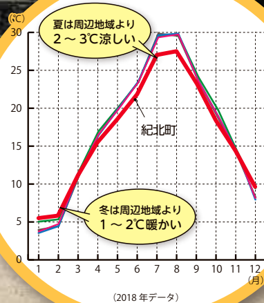
気温の平均値グラフ
