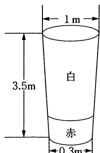
図1 吹流し
