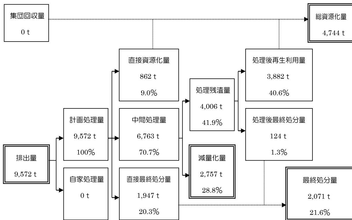
図 1 - 3 一般廃棄物の処理状況フロー（紀北町）
